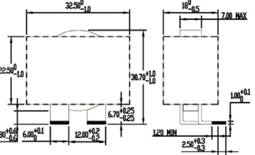
PQ3218-6R0-50-T - 6.0 \mu H
